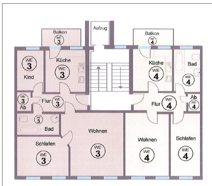
Grundriss Wohnung Nr. 3, ohne Maßstab
